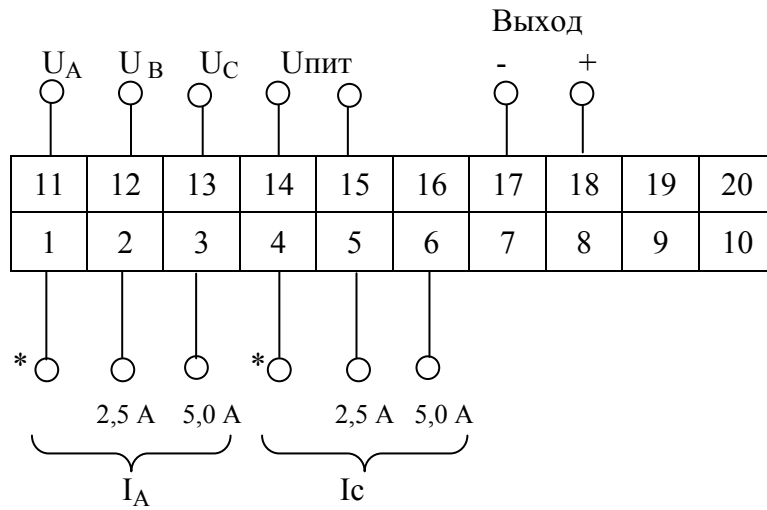
Рисунок А.2 – Схема подключения ИП Е 859/2ЭС, Е 859/4ЭС, Е 859/5ЭС
