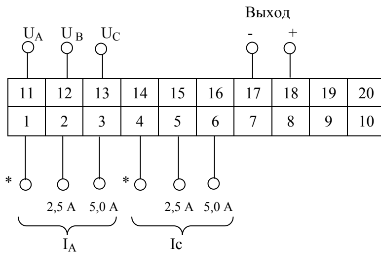
Рисунок А.3 – Схема подключения ИП Е 859/1ЭС, Е 859/3ЭС, Е 859/6ЭС
